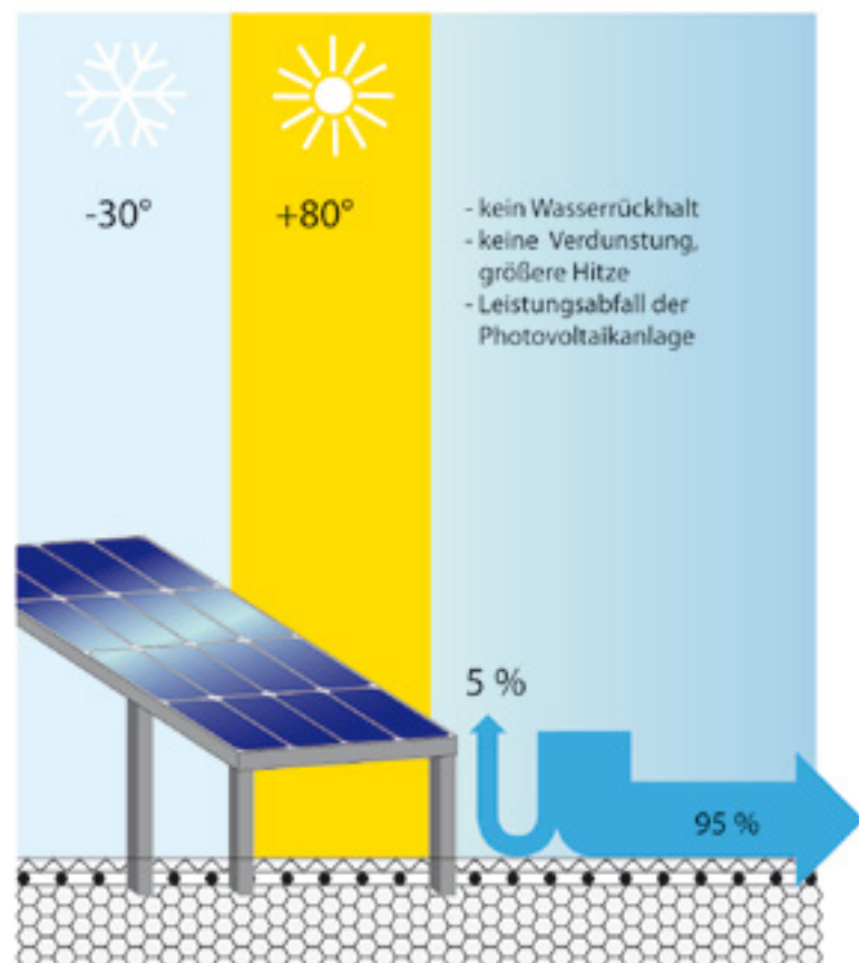
Photovoltaikanlage in der Dachkonstruktion verankert, ohne Dachbegrünung.
