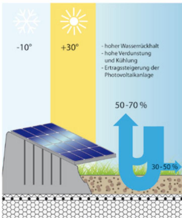
Kombination Photovoltaik mit Dachbegrünung. Auflastgehaltene System „SolarGrünDach“.
